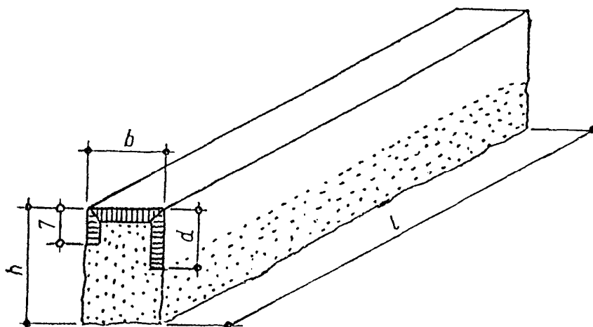
Rys. 4. Krawężnik najazdowy rodzaju B
