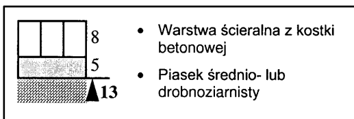
4. Nawierzchnia ścieżek rowerowych
