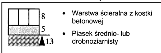
5. Nawierzchnia przeznaczona do postoju pojazdów i jezdni manewrowej (m.in. na parkingu)
