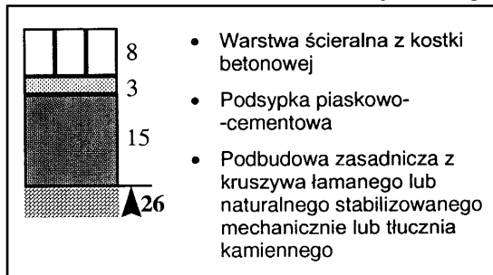
5. Nawierzchnia przeznaczona do postoju pojazdów i jezdni manewrowej (m.in. na parkingu)
