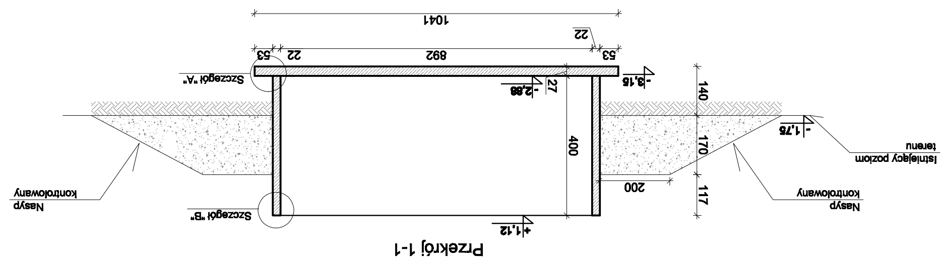
ZBIORNIK O ŚREDNICY 8,92m - WYKONAĆ 1SZT.
